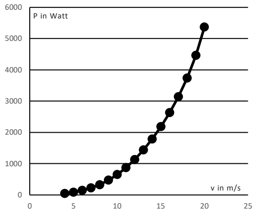
Leistungskurve AIR.5 Windturbine:
